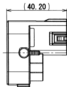
SEC. A-A
