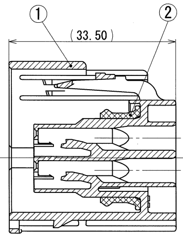
SEC. A-A
