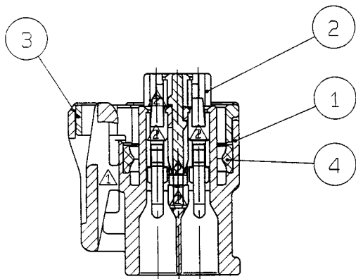
SEC. A-A
