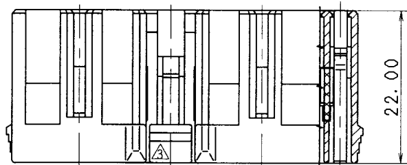
SEC. A-A
