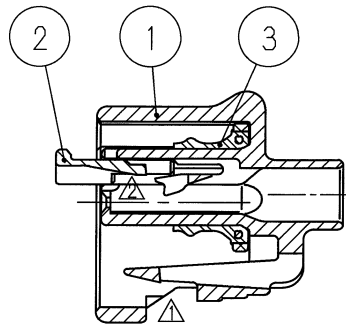
SEC. A-A
