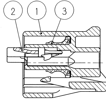
SEC. A-A
