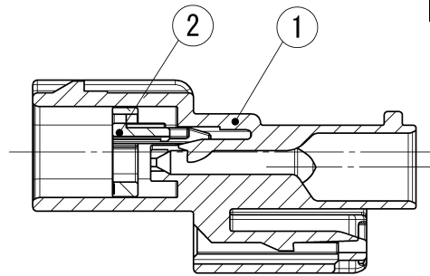
SEC. A-A
