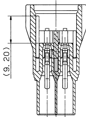
SEC. A-A
