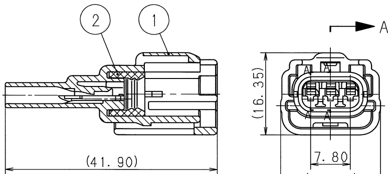
SEC. A-A
