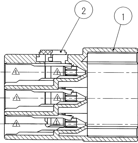
SEC. A-A
