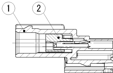
SEC. A-A
