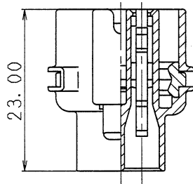
SEC. A-A
