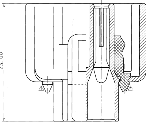
SEC. A-A
