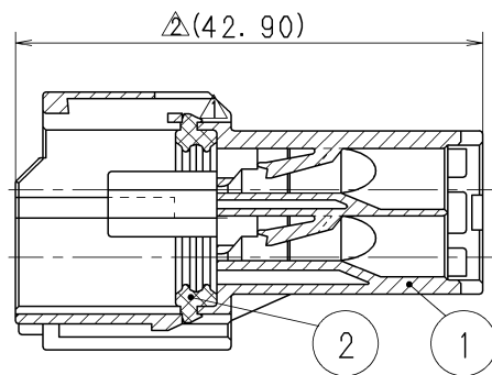
SEC. A-A
