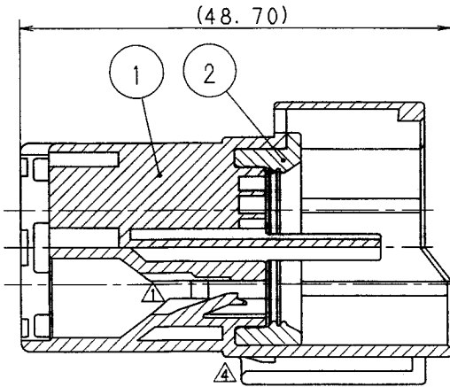
SEC. A-A
