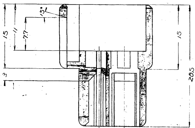
A-A断面图
