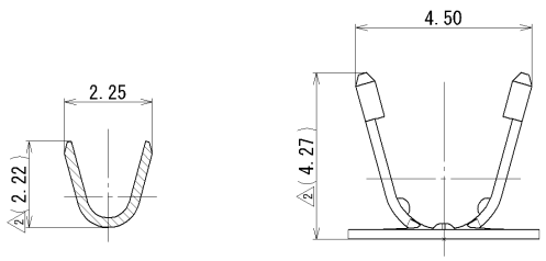
SEC. A-A
