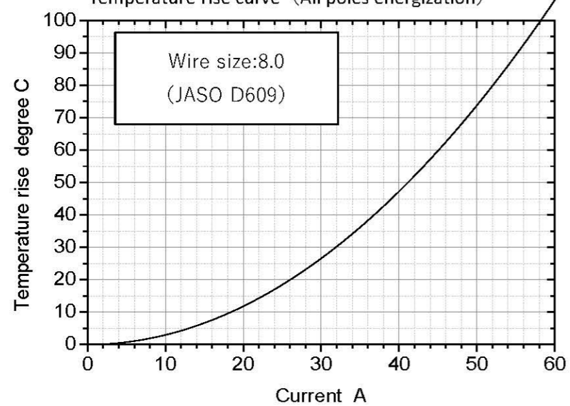
温度上昇曲線 (全極通電)
