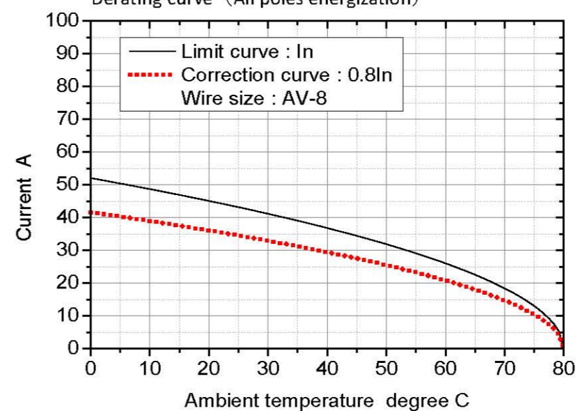
軽減曲線 (全極通電)
