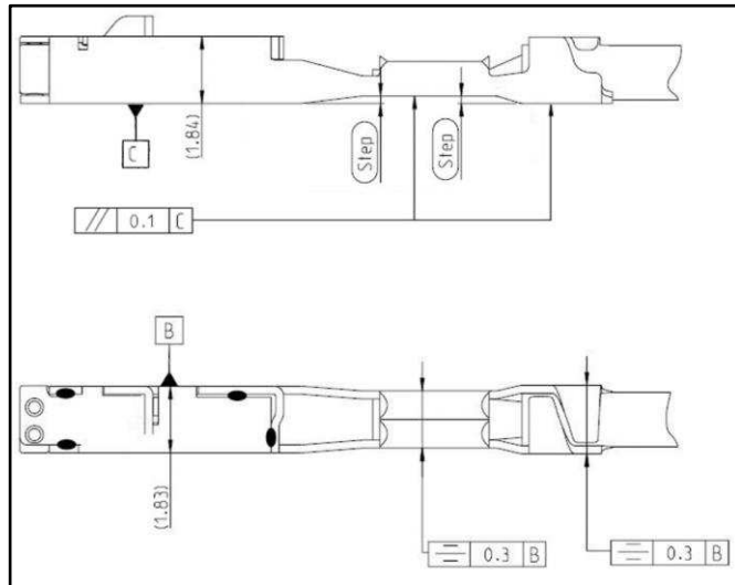
Fig. / Abb. 4: Shape and Position Tolerances / Form- und Lagetoleranzen
